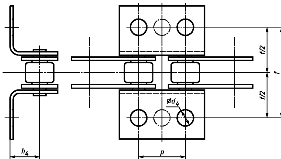
б — на внутреннем звене
