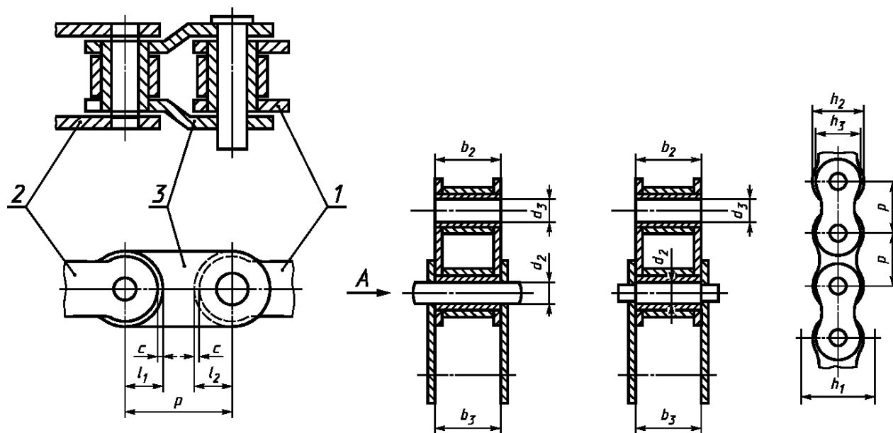
a — звено с изогнутыми пластинами b — сечение с гладкими валиками в — сечение цепи со ступенчатыми валиками
