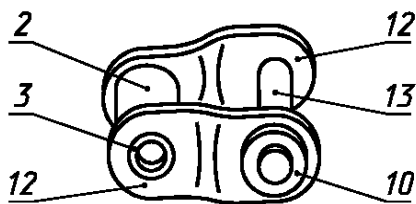
е — переходное звено однорядное
