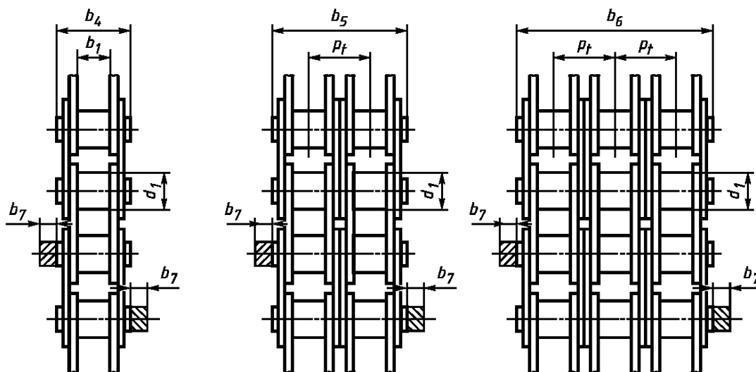
г — однорядная цепь д — двухрядная цепь е — трехрядная цепь
