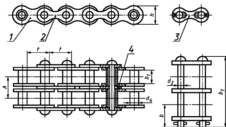
Рисунок 5 — Цепь типа ПВ
