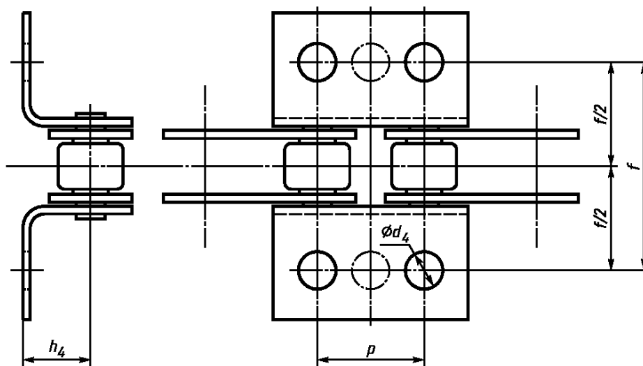
а — на наружном звене
